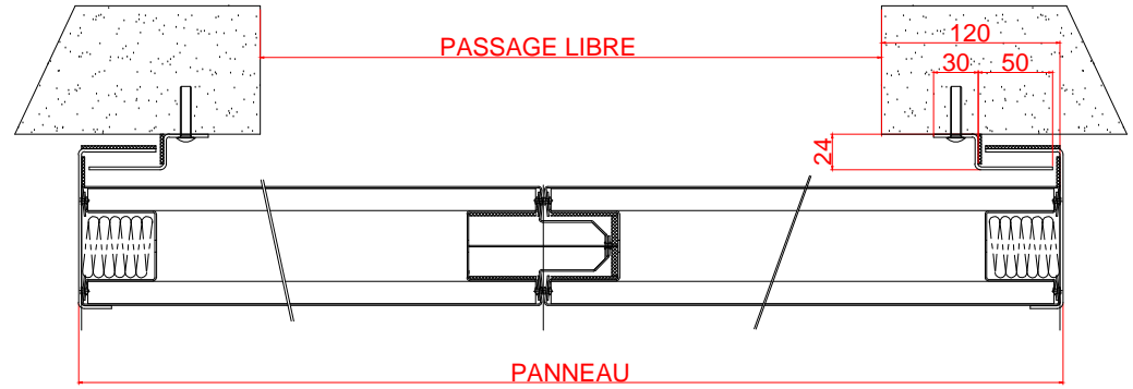
COUPE HORIZONTALE STANDARD
